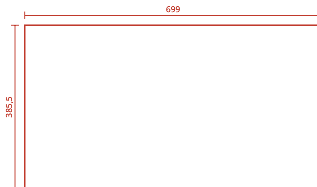
Rückwand Abwicklung
