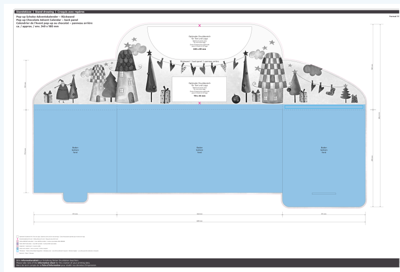
KSW-Standskizze Rückwand mit den Logo-Flächen (weiß) – verkleinert
